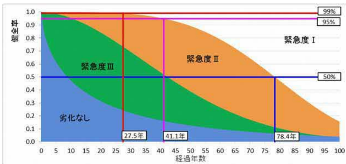
図 7-2-2 P-F 曲線による管理区分と目標基準までの年数 (劣化なし～緊急度 )
