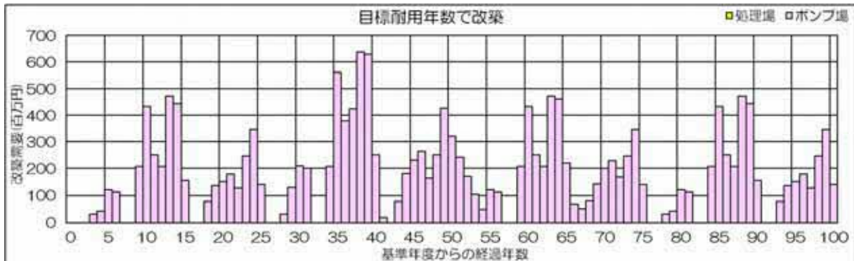
図 6-3-2 ポンプ場・処理場施設のシナリオ別改築需要
